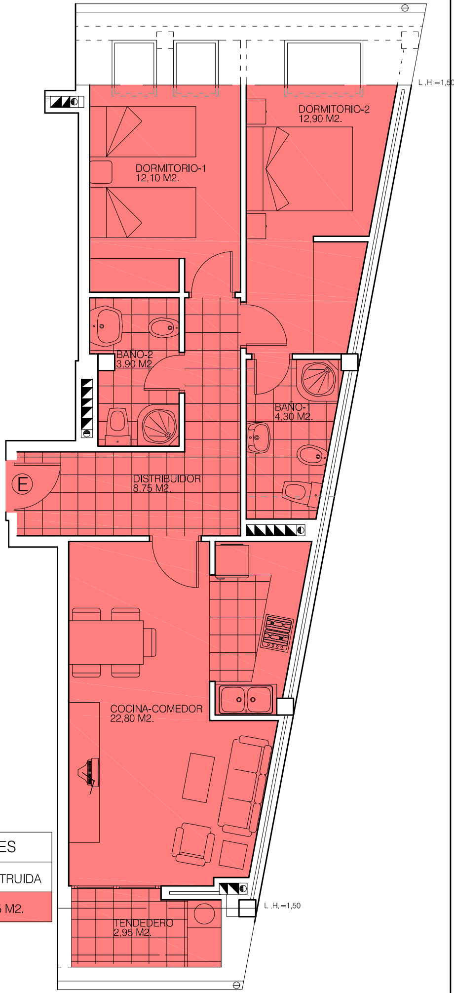
PLANTA BAJO CUBIERTA, VIVIENDA TIPO "E"
